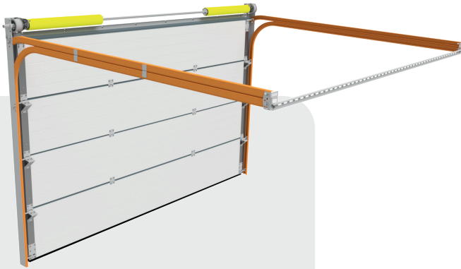
Rail de roulement F - Hauteur du linteau min. 200 mm
