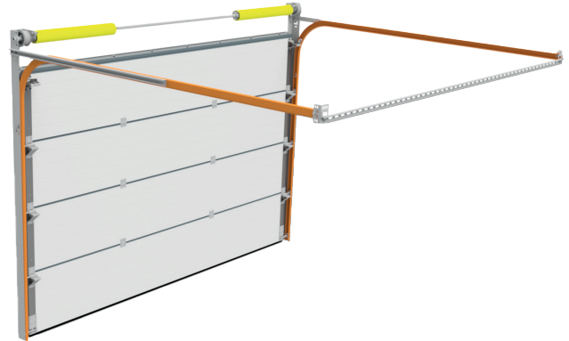
Rail de roulement S - Hauteur de linteau min.
