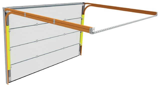
Rail de roulement Z - hauteur de linteau min. 80 mm (manuel) ou 120 mm (automatique)
