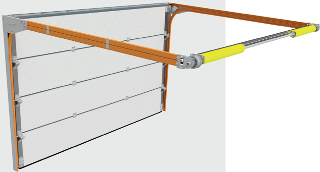
Rail de roulement R - Hauteur de linteau min. 80 mm (manuel) ou 120 mm (automatique)
